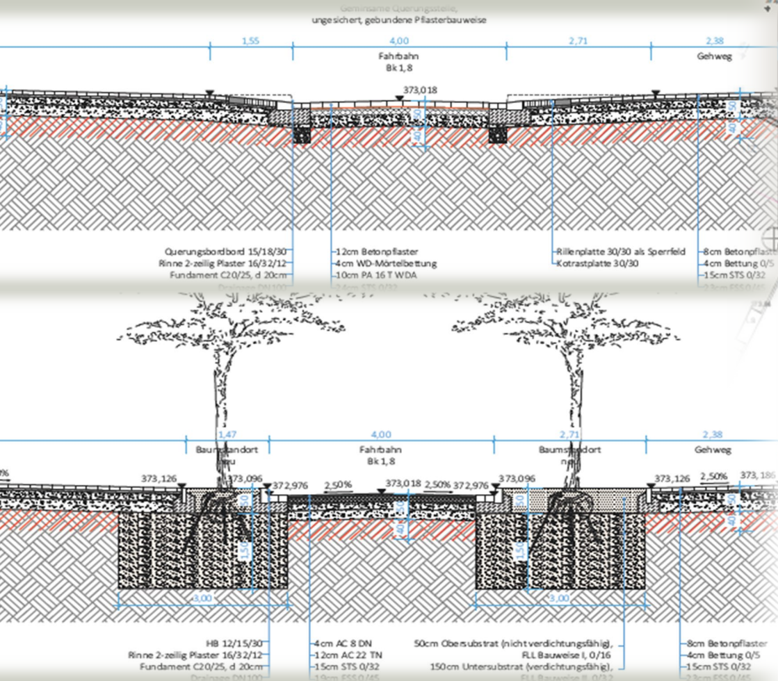
Querschnitte
