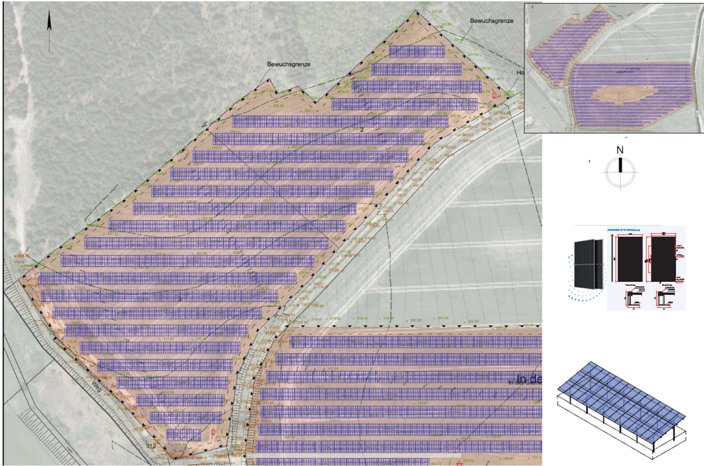
Schnitt Fläche Nord - M= 1:750
